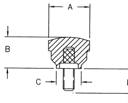
THREADED STUD
